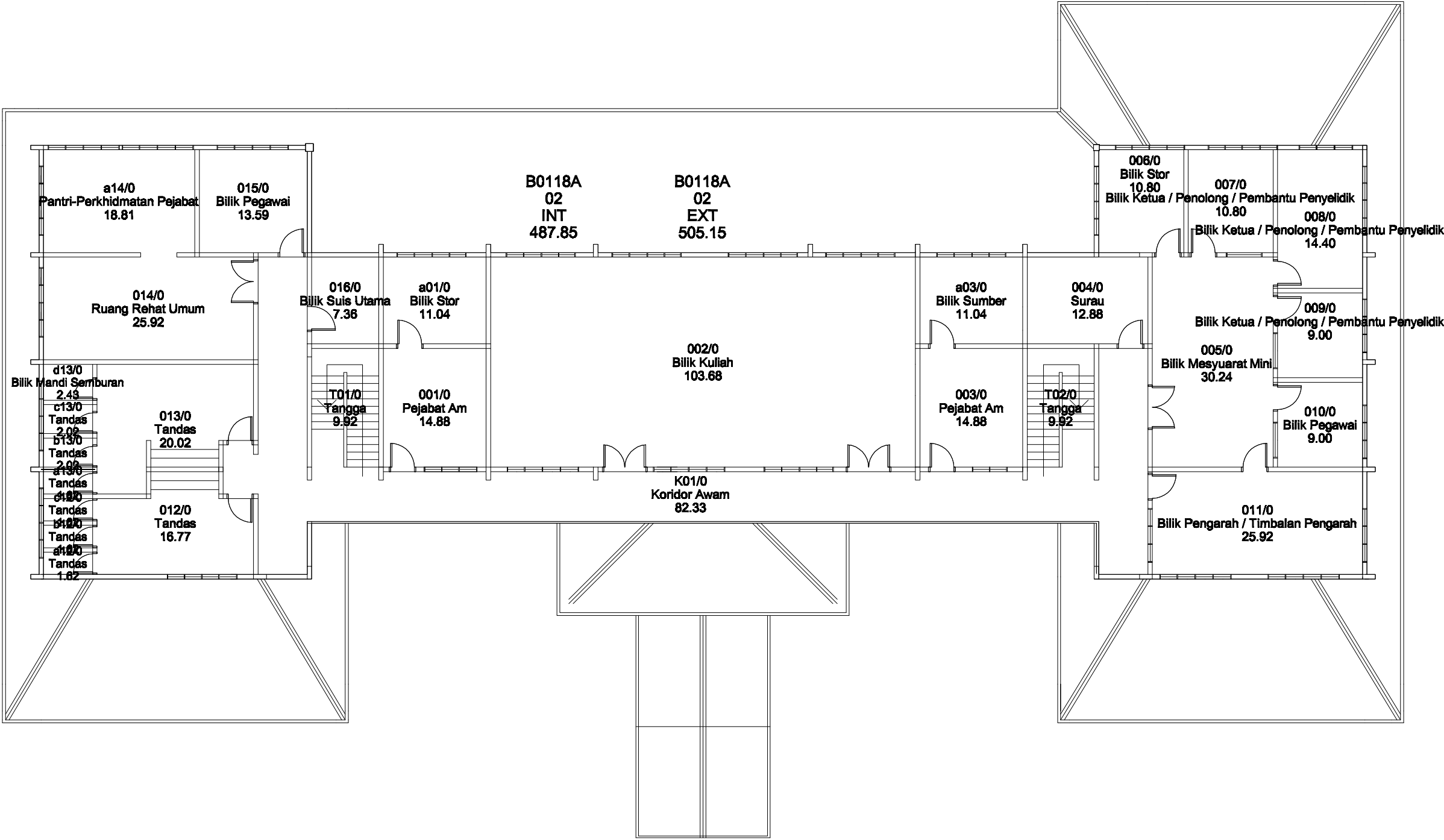
MARKAS PALAPES - ARAS 2 SCALE : 1:150
